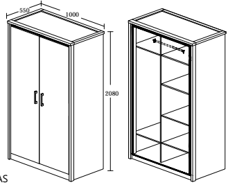
ELIAS MODEL : WR 80183-S5V-P ITEM : KLEERKAST-ARMOIRE 2 D/P / 2 DOORS WARDROBE PRODUCT SIZE : L 100 X D 55 X H 208cm
