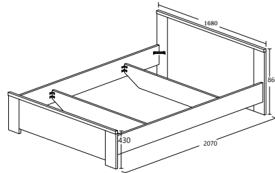
ELIAS MODEL : BED 54-6379C-S5V ITEM : BED - LIT 160 / BED 160 PRODUCT SIZE : L 168 X D 207 X H 86cm MS: L 160 X D 200cm
