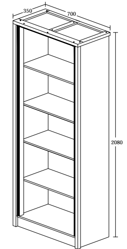
ELIAS MODEL : BC 70100-S5V-P ITEM : BOEKENREK / ETAGERE / BOOKCASE PRODUCT SIZE : L 70 X D 35 X H 208cm
