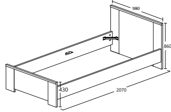
ELIAS MODEL : BED 54-3679C-S5V ITEM : BED - LIT 90 / BED 90 PRODUCT SIZE : L 98 X D 207 X H 86cm MS: L 90 X D 200cm
