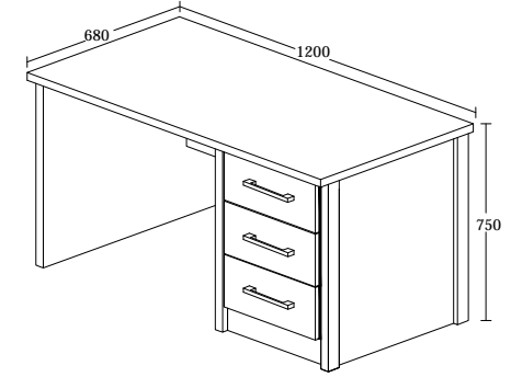
ELIAS MODEL : WT 2016-S5V-P ITEM : BUREEL - BUREAU 120 / WRITING TABLE 120 PRODUCT SIZE : L 120 X D 68 X H 75cm
