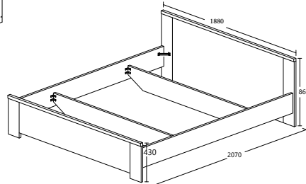
ELIAS MODEL : BED 54-7179C-S5V ITEM : BED - LIT 180 / BED 180 PRODUCT SIZE : L 188 X D 207 X H 86cm MS: L 180 X D 200cm
