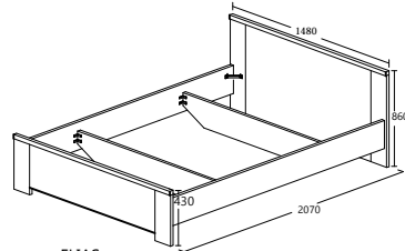
ELIAS MODEL : BED 54-5579C-S5V ITEM : BED - LIT 140 / BED 140 PRODUCT SIZE : L 148 X D 207 X H 86cm MS: L 140 X D 200cm
