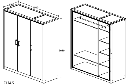
ELIAS MODEL : WR 80184-S5V-P ITEM : KLEERKAST-ARMOIRE 3 D/P / 3 DOORS WARDROBE PRODUCT SIZE : L 150 X D 55 X H 208cm
