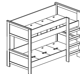
ELINE MODEL : BED 71-S5V ITEM : BUNKER BED L 108.2 X D 207.5 X H 178cm
