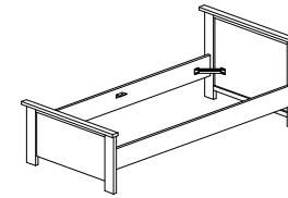
ELINE MODEL : BED 70-3679C-S5V ITEM : BED-LIT 90 L 209 X D 108 X H 95cm M/S: L90 X 200 cm
