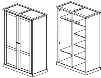
ELINE MODEL : WR 80230-S5V ITEM : KLEERKAST / ARMOIRE 2D/P / 2 DOORS WARDROBE L 118 X D 58 X H 214cm
