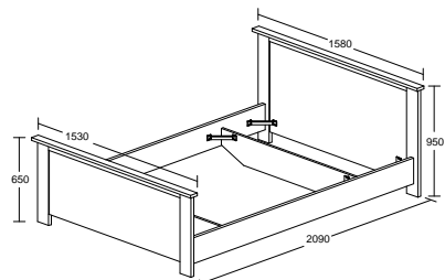
ELLA MODEL : BED 27-5579C-S5V ITEM : BED - LIT 140 L 209 X D 158 X H 95 cm M/S : L140 X 200 cm
