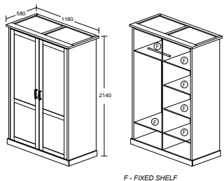
ELLA MODEL : WR 80096-S5V ITEM : KLEERKAST / ARMOIRE 2D/P / 2 DOORS WARDROBE L 118 X D 58 X H 214 cm
