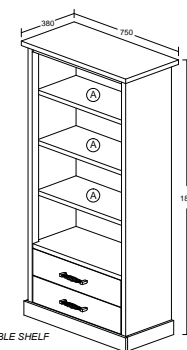
ELLA MODEL : BC 70072-S5V ITEM : BOEKENREK / BIBLIOTHEQUE / 2 DRAWERS BOOKCASE L 75 X D 38 X H 185 cm
