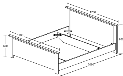
ELLA MODEL : BED 27-6379C-S5V ITEM : BED - LIT 160 L 209 X D 178 X H 95 cm M/S : L160 X 200 cm
