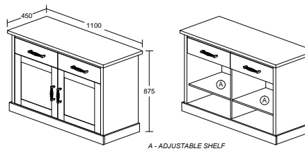
ELLA MODEL : DTC 333-S5V ITEM : COMMODE 2 LADEN 2 D/P / CHEST L 110 X D 45 X H 87.5 cm
