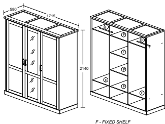
ELLA WR 80097-1M-S5SV ITEM : KLEERKAST / ARMOIRE 3D/P / 3 DOORS WARDROBE WITH 1 MIRROR L 171.5 X D 58 X H 214 cm
