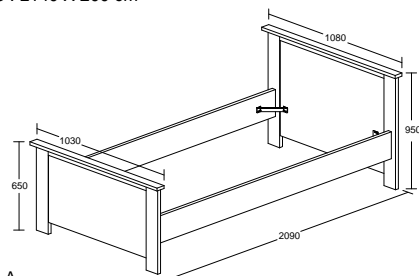
ELLA MODEL : BED 27-3679C-S5V ITEM : BED - LIT 90 L 209 X D 108 X H 95 cm M/S : L90 X 200 cm
