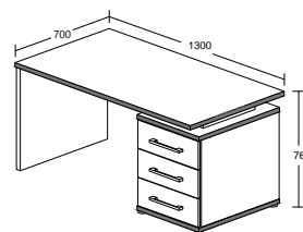
ELLEN MODEL : WT 2025-S5V ITEM : WRITING TABLE L 130 X D 70 X H 76.2cm
