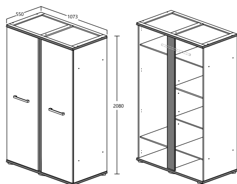
ELLEN MODEL : WR 80207-S5V ITEM : 2 DOORS WARDROBE L 107.3 X D 55 X H 208cm
