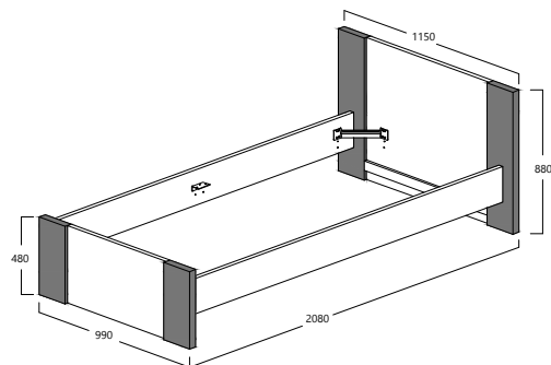
ELLEN MODEL : BED 58-3679C-S5V ITEM : BED L 208 X D 115 X H 88cm
