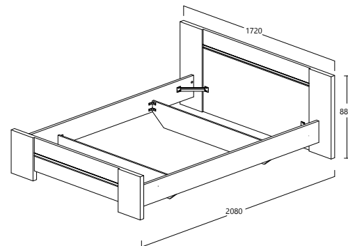
ERWIN MODEL : BED 69-5579C-FO-S5V ITEM : BED-LIT 140 L 172 X D 208 X H 88cm
