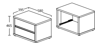
ERWIN MODEL : BST 55001-FO-S5V ITEM : NACHTTAFEL / TABLE DE UNIT / NIGHT STAND L 58 X D 39.5 X H 46.5cm
