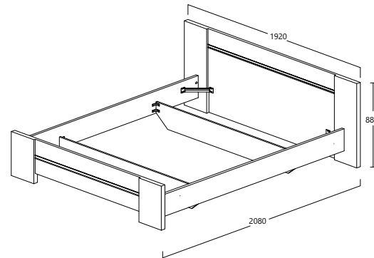
ERWIN MODEL : BED 69-6379C-FO-S5V ITEM : BED-LIT 160 L 192 X D 208 X H 88cm
