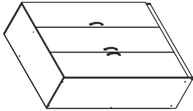
Item : KLEERKAST / GARDE ROBE 80 Model : DN WAR 200104 W800 x D500 x H1800mm
