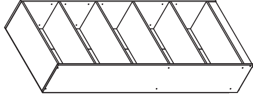
Item : BOEKENREK / ETAGERE Model : DN STC 201450 W700 x D295 x H1800mm
