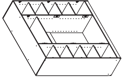
Item : KLEERKAST / GARDE ROBE 120 Model : DN WAR 300103 W1200 x D500 x H1800mm
