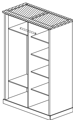
EMMA MODEL : WR 80145-S5V ITEM : KLEERKAST / ARMOIRE 2D/P / 2 DOORS WARDROBE L 118 X D 58 X H214cm
