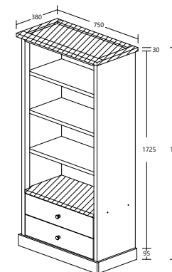
EMMA MODEL : BC 70086-S5V ITEM : BOEKENREK / BIBLIOTHEQUE / 2 DRAWERS BOOKCASE L 75 X D 38 X H 185cm
