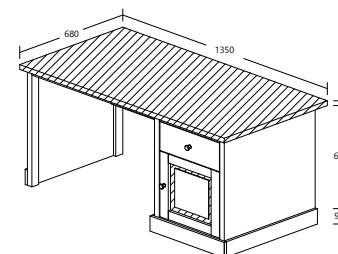
EMMA MODEL : WT 2006-S5V ITEM : BUREEL / BUREAU / WRITING TABLE L 135 X D 68 X H 75cm
