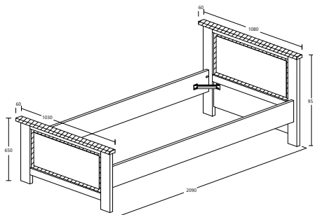
EMMA MODEL : BED 35-3679C-S5V ITEM : BED-LIT 90 L 209 X D 108 X H95cm M/S : L 90 X 200cm
