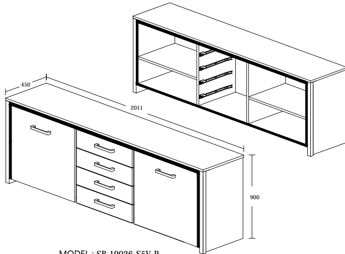
MODEL : SB 19026-S5V-P ITEM : ELIAS DRESSOIR 211 / SIDEBOARD COLOR : NEW GREY OAK + BLACK LINE PRODUCT SIZE : L 201.1 x D 45 x H 90cm
