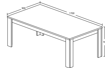
MODEL : DS 019-S5V-P ITEM : EETTAFEL / TABLE 170 / DINING TABLE 170 COLOR : NEW GREY OAK PRODUCT SIZE : L 170 X D 90 X H 76cm
