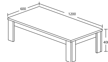
MODEL : CT 15035-S5V-P ITEM : SALONTAFEL / TABLE BASSE 120 / SOFA TABLE 120 COLOR : NEW GREY OAK PRODUCT SIZE : L 120 X D 60 X H40cm
