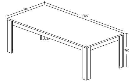
MODEL : DS 020-S5V-P ITEM : EETTAFEL / TABLE 190 / DINING TABLE 190 COLOR : NEW GREY OAK PRODUCT SIZE : L 190 X D 90 X H 76cm
