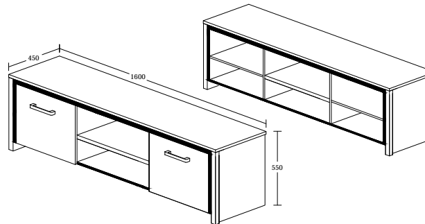
MODEL : EC 60155-S5V-P ITEM : ELIAS TV 160 / TV CABINET COLOR : NEW GREY OAK + BLACK LINE PRODUCT SIZE : L 160 x D 45 x H 55cm
