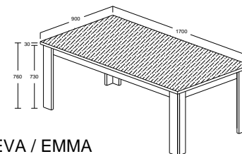
EMILY / EVA / EMMA MODEL : 1236-S5V ITEM : EETTAFEL / TABLE / DINING TABLE 190 L 190 X D 90 X H 76cm
