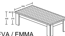
EMILY / EVA / EMMA MODEL : 1235-S5V ITEM : SALONTAFEL / TABLE BASSE / SOFA TABLE 120 L 120 X D 60 X H 40cm
