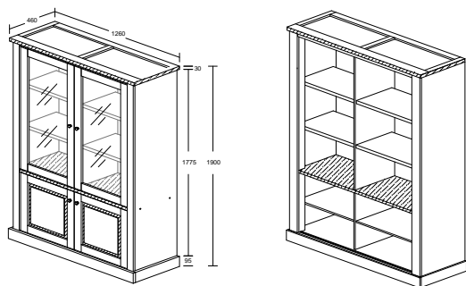
EMMA MODEL : BC 70083-G-S5V ITEM : GLASKAST / ARGENTIER / GLASS CABINET L 126 X D 46 X H 190cm
