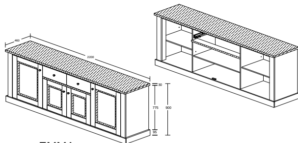
EMMA MODEL : SB 19020-S5V ITEM : DRESSOIR 220 / SIDE BOARD L 220 X D 46 X H 90 cm
