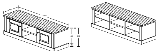
EMMA MODEL : EC 60122-S5V ITEM : TV KAST / MEUBLE TV / TV CABINET L 155 X D 46 X H 54.8cm
