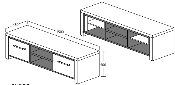
ENSOR MODEL : EC 60178-S5V ITEM : TV CABINET L 150 X D 45 X H 50cm
